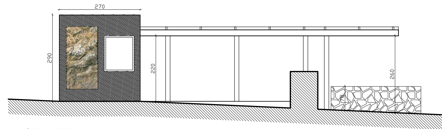
VISTA LATERAL
