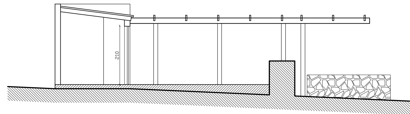
CORTE AA
